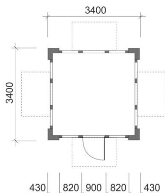
План M1:100
