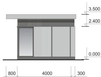
Вид сбоку M1:100
