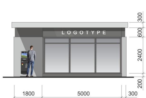
Вид спереди M1:100
