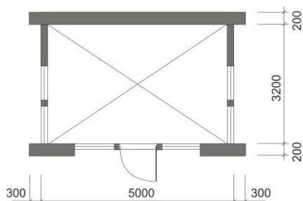
План M1:100
