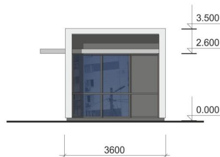
Вид сбоку M1:100
