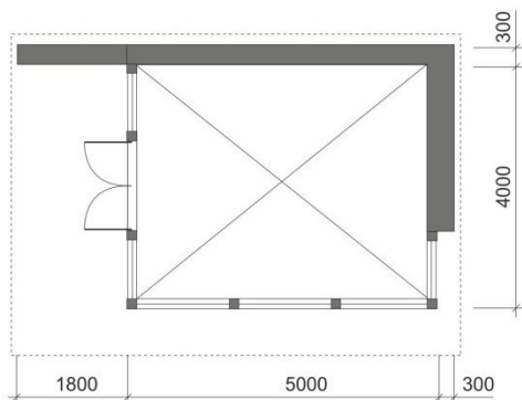
План M1:100
