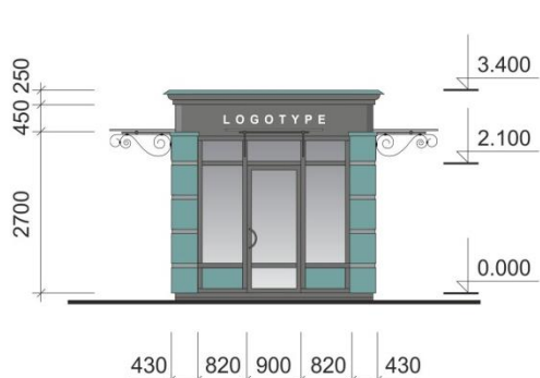
Вид спереди M1:100
