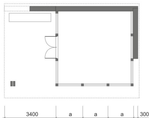
План М1:100
