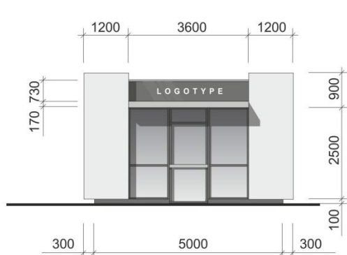
Вид спереди M1:100
