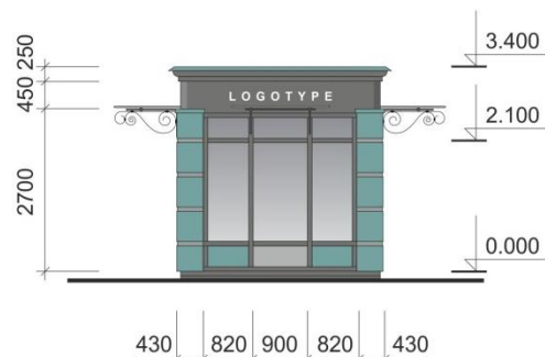
Вид сбоку M1:100
